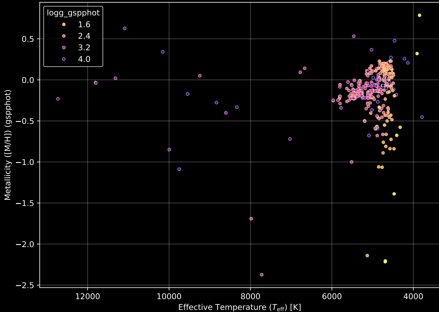
APOGEE DR17 Field: [191-08] Stellar Population Parameters (n= 304)
